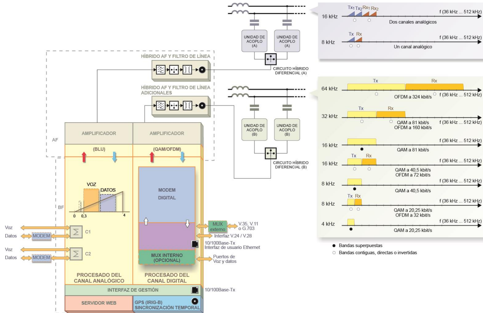
FIGURA 2 Arquitectura básica del terminal OPU-1 de 20 y 40 W con filtros adicionales (ejemplos de configuración)
