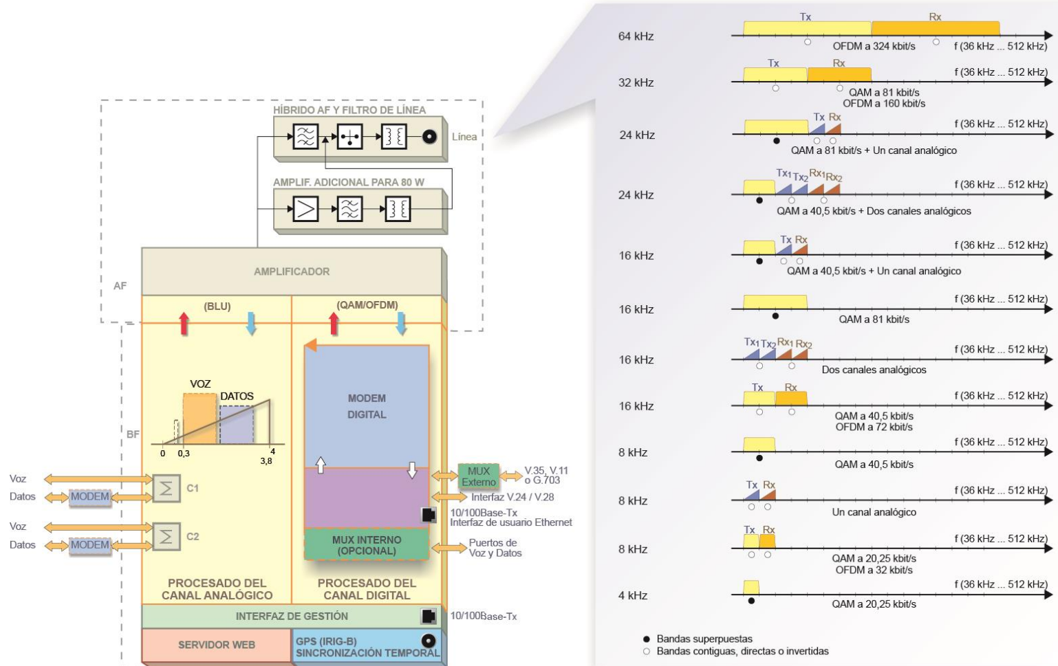
FIGURA 1 Arquitectura básica del terminal OPU-1 de 20, 40 y 80 W (ejemplos de configuración)
