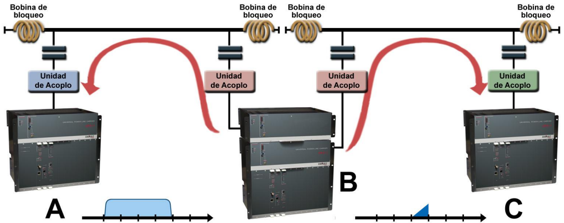
FIGURA 5 Dos equipos de OP independientes en un único panel
