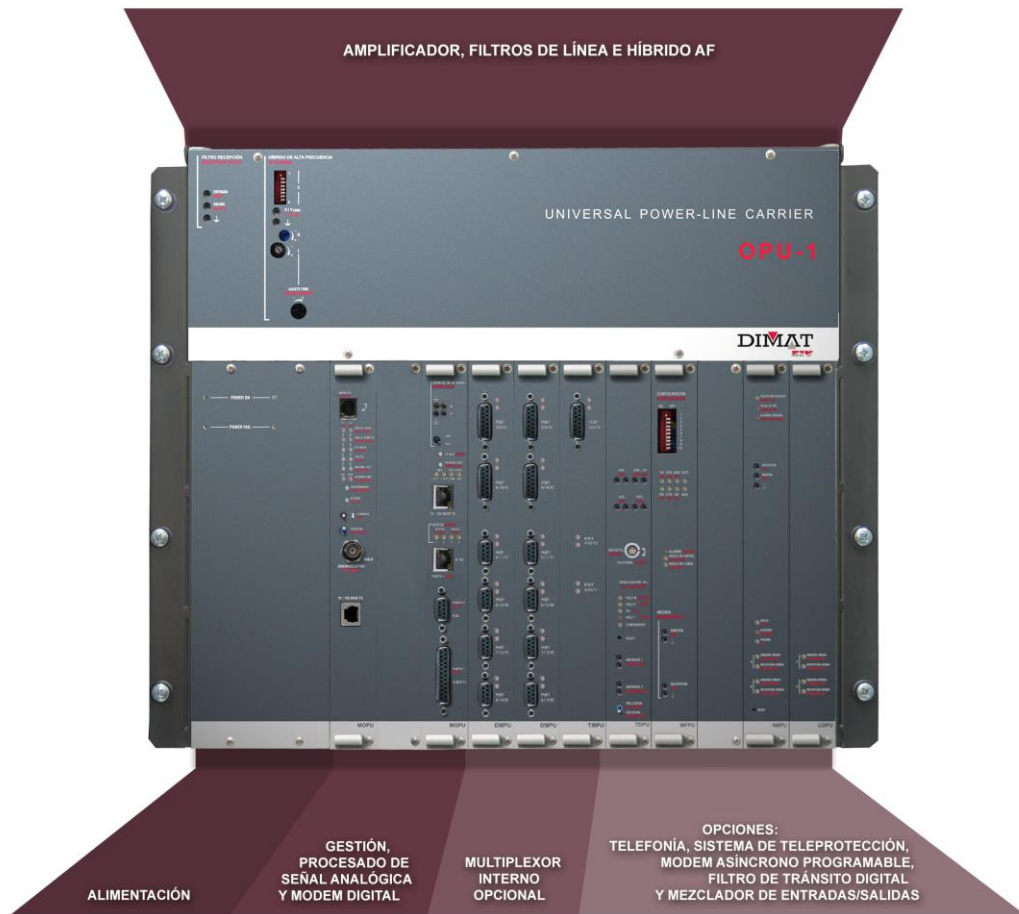
FIGURA 15 Disposición de módulos
